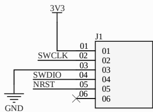
Header 6
